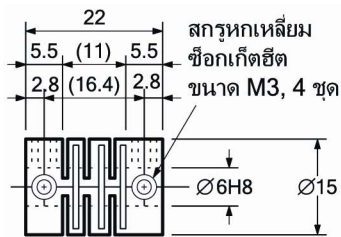
E69-C06B
